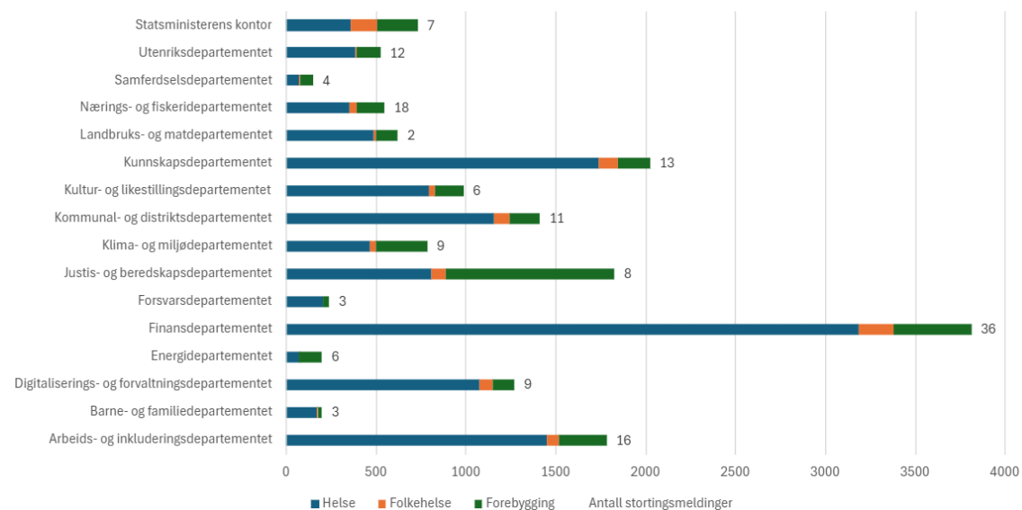
Forordningen av søkeord i departementenes Stortingsmeldinger (2019-2024)
